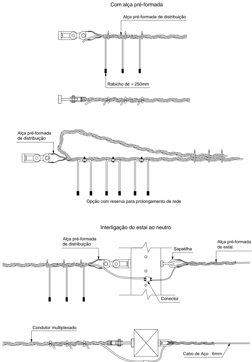
Figura 40 – Amarrações e ligações – Estrutura secundária – Fim de rede
