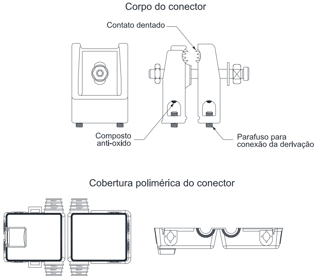
Figura 60 – Conexões e emendas – Conector de múltiplas derivações
