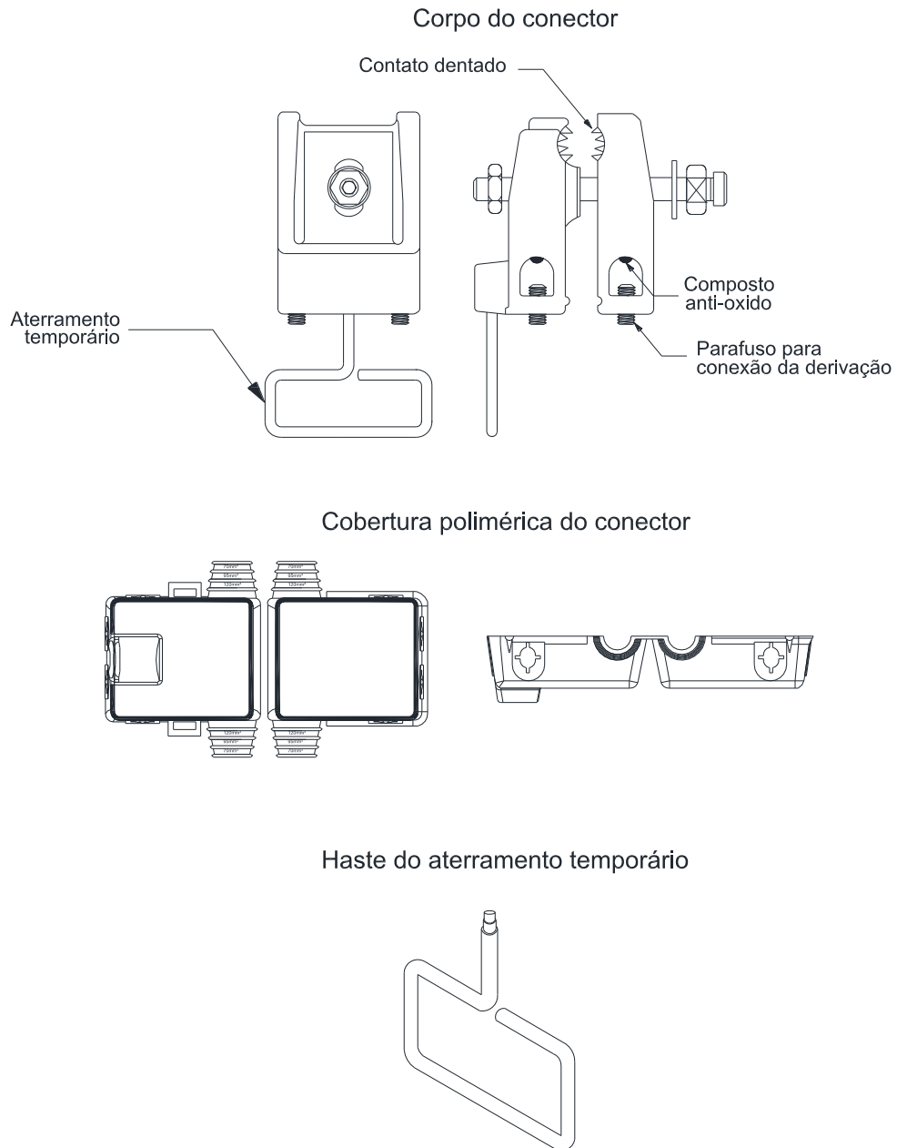
Figura 61 – Conexões e emendas – Conector de múltiplas derivações com aterramento
