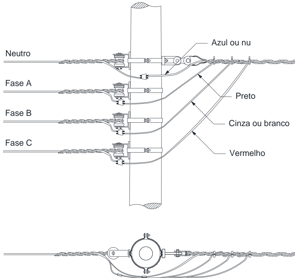
Figura 22 – Estrutura transição rede nua / rede isolada – S3 – S13
