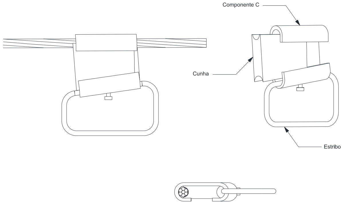
Figura 56 – Conexões – Conector cunha com estribo
