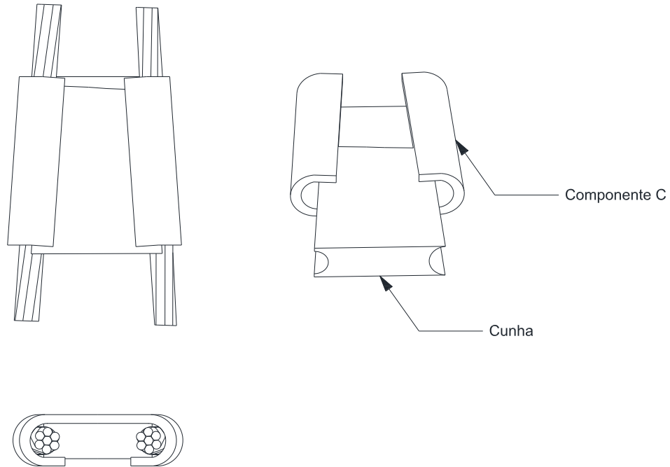
Figura 55 – Conexões – Conector cunha
