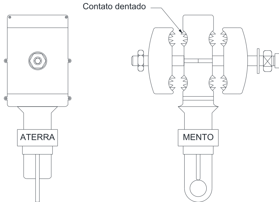
Figura 62 – Conexões e emendas – Conector de aterramento temporário
