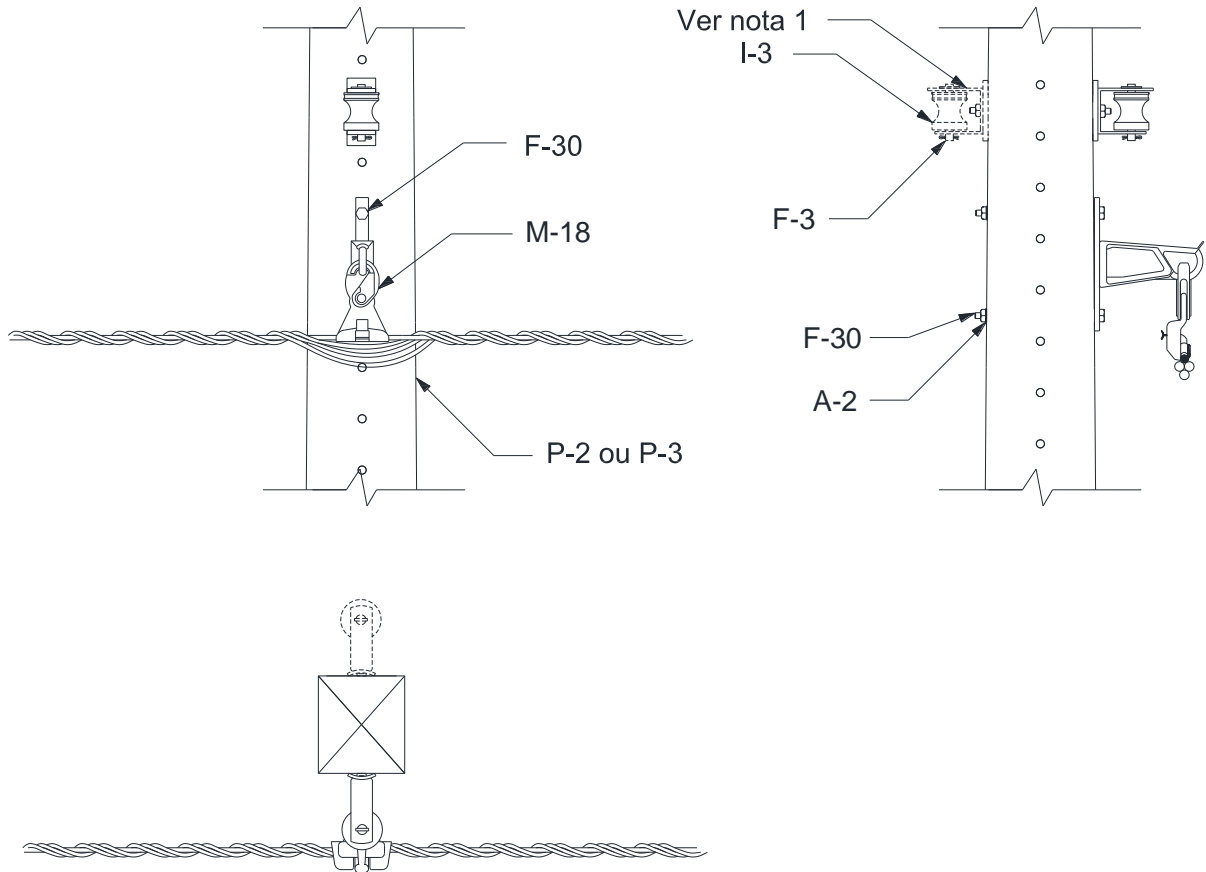
Figura 11 – Estruturas tangentes – S11 – Poste de concreto de seção DT ou madeira
