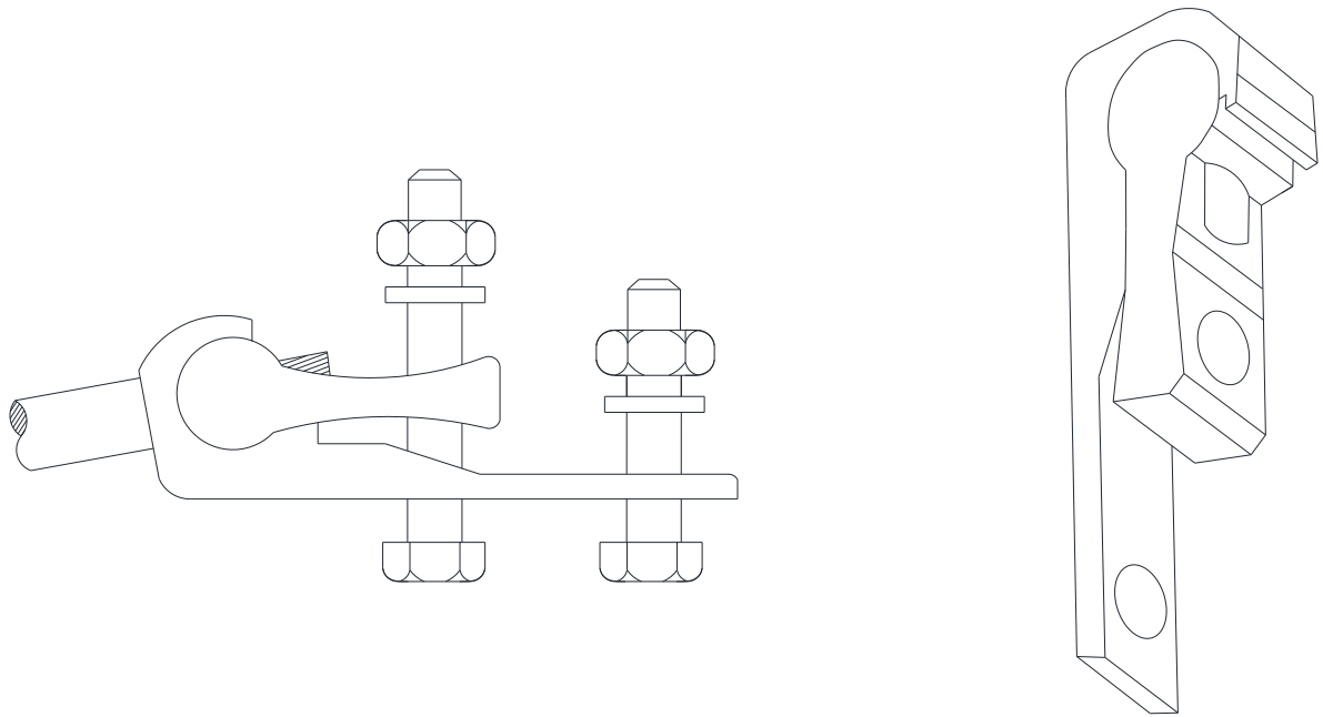
Figura 59 – Conexões e emendas – Conector terminal de estrangulamento
