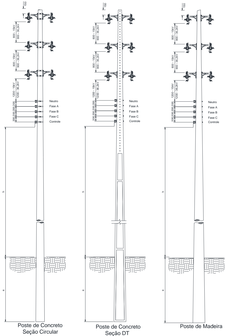
Figura 13 – Afastamentos mínimos – Estruturas trifásicas tangentes
