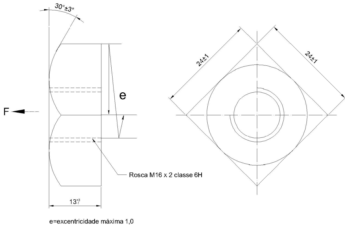
Figura 115 - Porca quadrada
