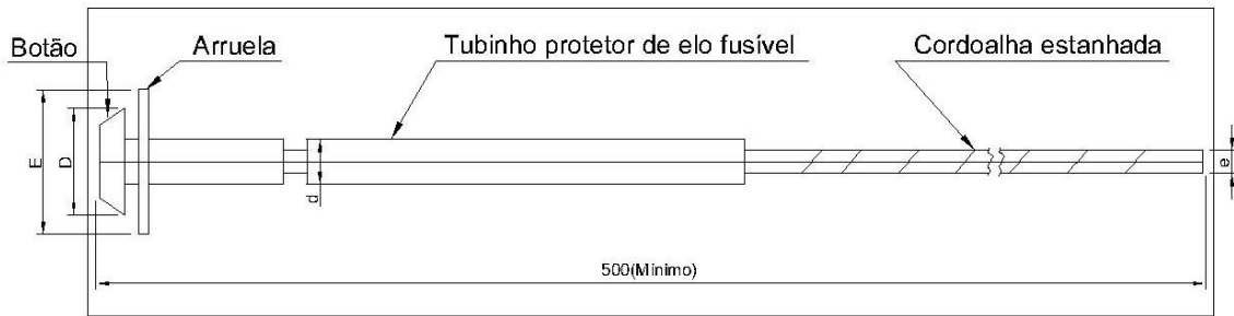
Figura 67 - Elo fusível
