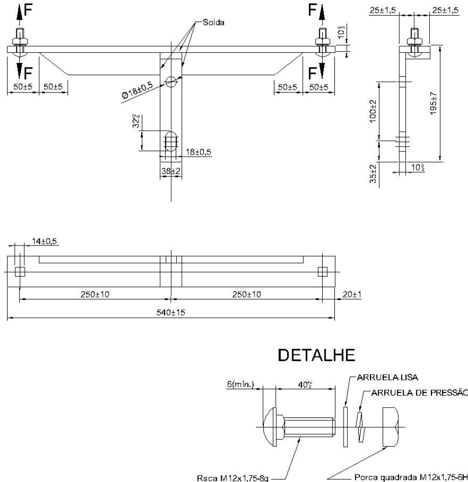
Figura 134 - Suporte T
