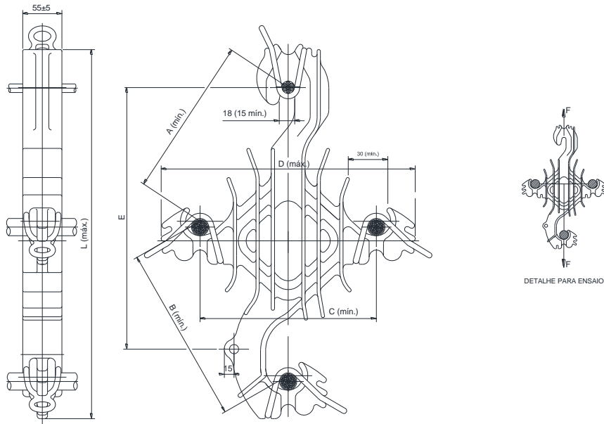
Figura 70 - Espaçador losangular
