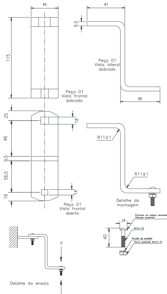
Figura 136 - Suporte Z
