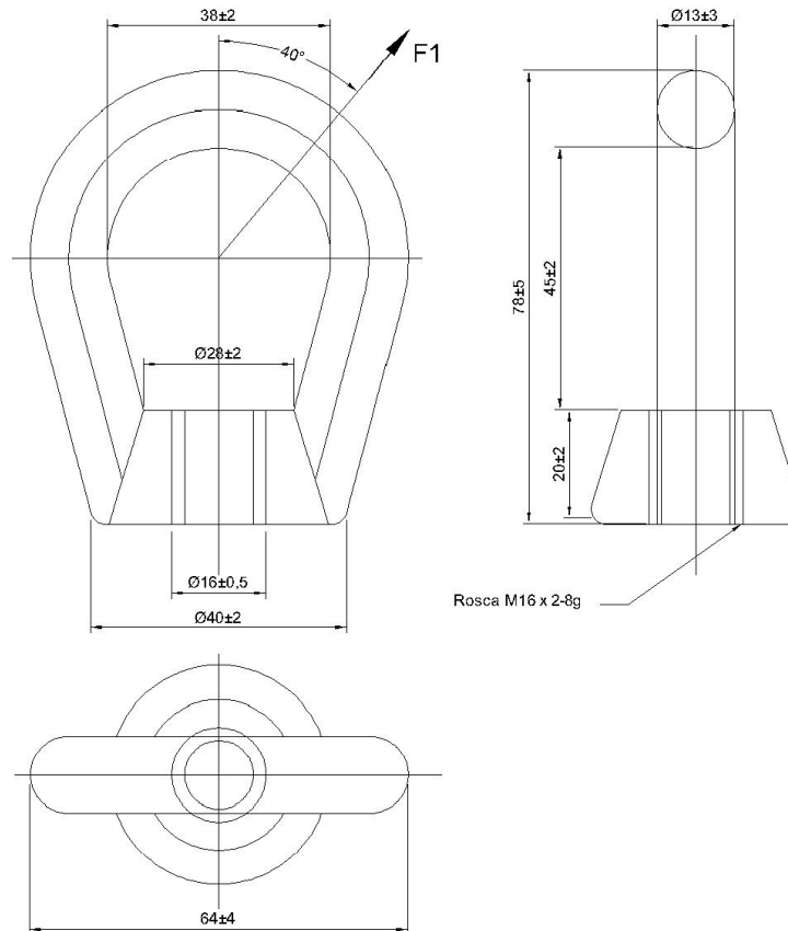
Figura 114 - Porca olhal
