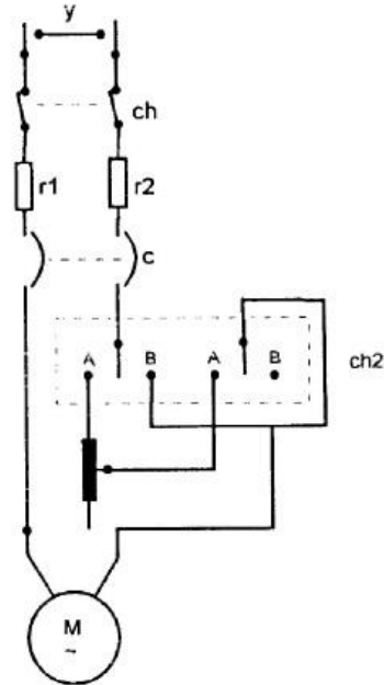
Figura 1 - Partida com chave compensadora
