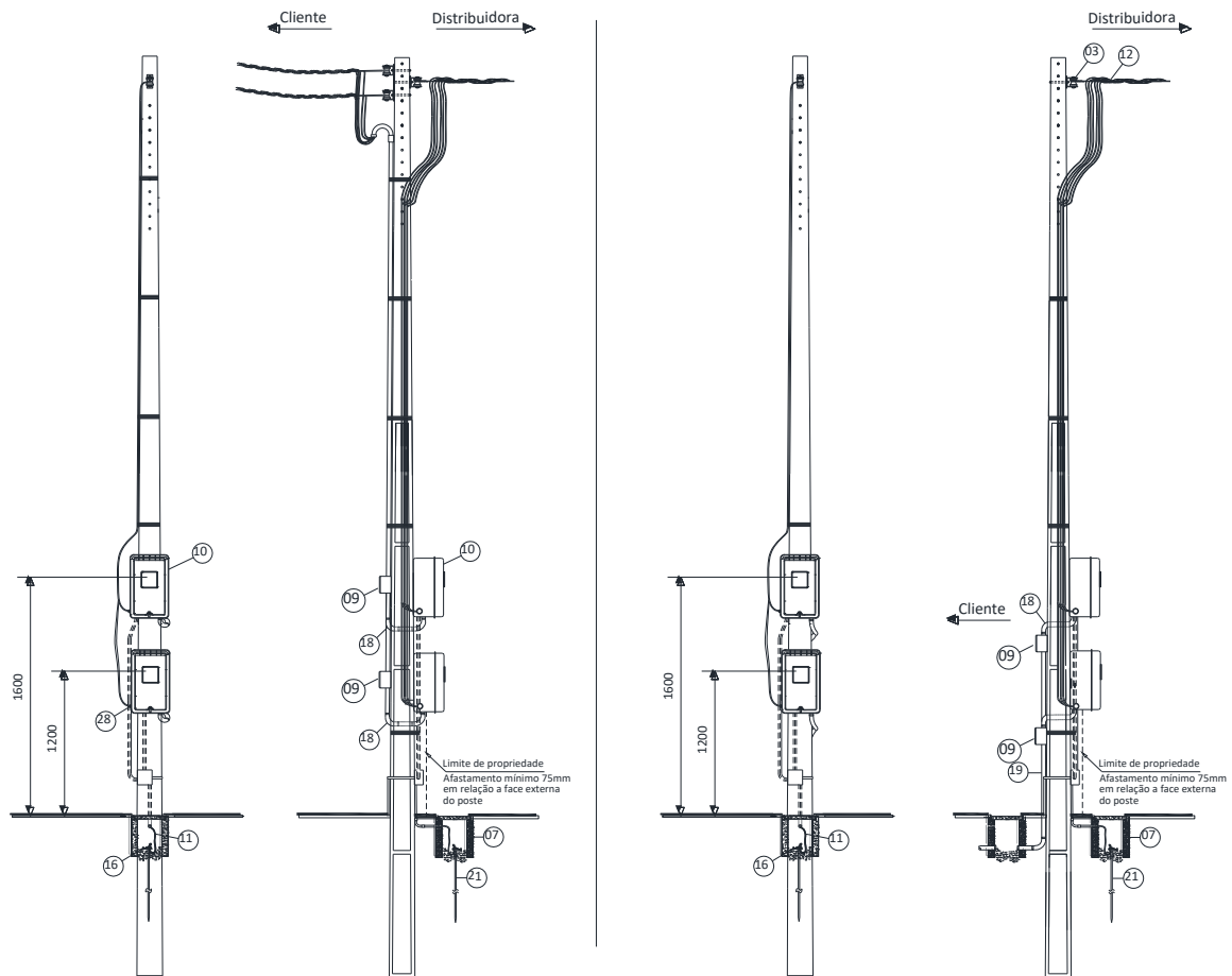
Saída Aérea
